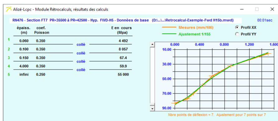
Module Retrocalculs- Ecran de comparaison entre bassins mesuré et rétrocalculé Option de calcul n°1 (algorithme de descente)
